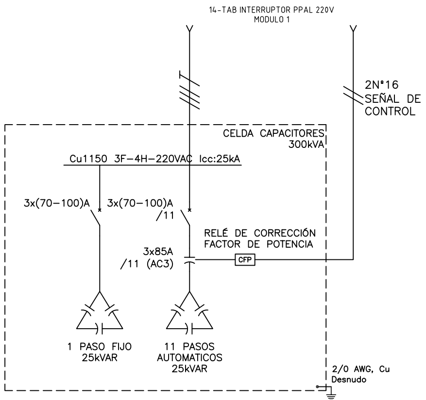
BANCO DE CAPACITORES DE 300KVAR, CON RELÉ DE 12 PASOS, CON 1 PASO FIJO Y 11 PASOS AUTOMÁTICOS DE 25kVAR EFÉCTIVOS A 220V, CON CONTACTOR AUXILIAR EN LA ENTRADA COMÚN DEL RELÉ PARA CONMUTACIÓN DE PASOS AUTOMÁTICOS
