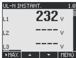
Figura 3-3 Visualización de la tensión medida con el tipo de conexión 1P2W
