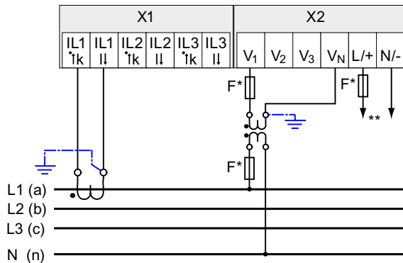
Figura 6-11 Tipo de conexión 3P4WB, con transformador de tensión, con un transformador de corriente
