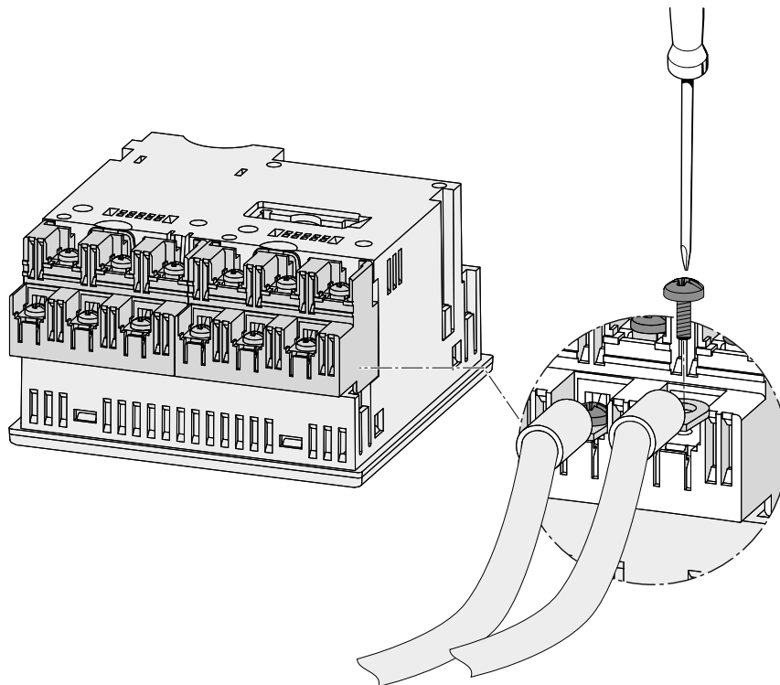
Figura 6-7 Conexión de los cables en las conexiones para terminales de ojal:
