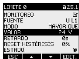
Figura 9-20 Parámetro ajustable "LÍMITE 0"
