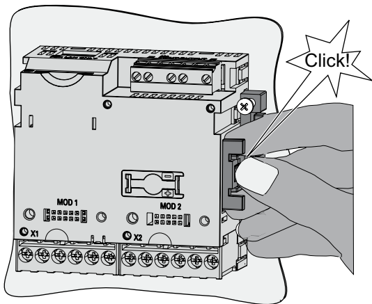
Paso de montaje C
